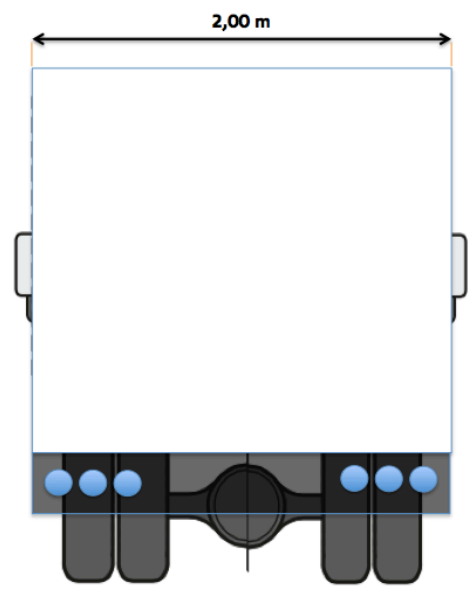
VUE ARRIÈRE
